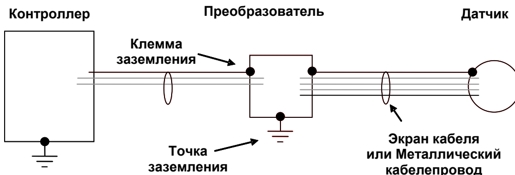
Рисунок 10. Заземление
