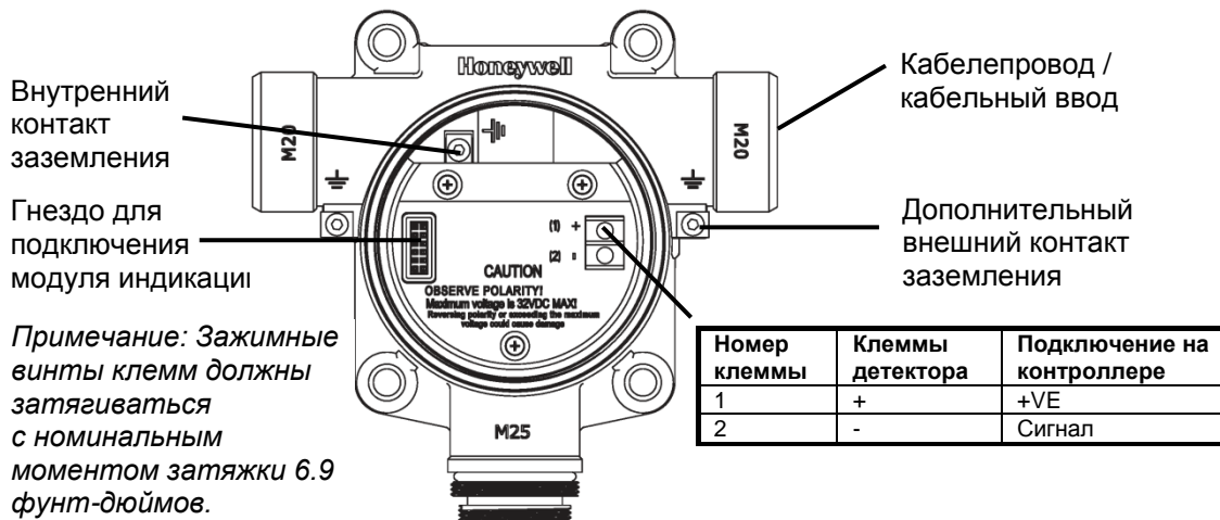
Рисунок 9. Контакты терминального модуля
