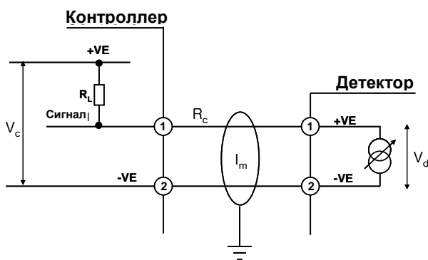
Рисунок 8. Монтажная электрическая схема, тип 2
