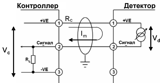
Рисунок 7. Монтажная электрическая схема, тип 1
